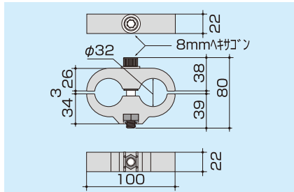
093-30 クランプ 300角用
