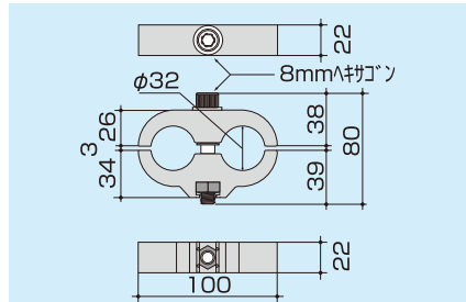
094-30 クランプ 200角用
