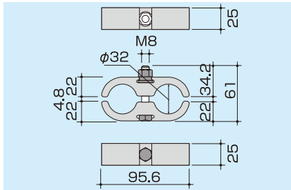
094-31 Cクランプ 200角・300角共用
