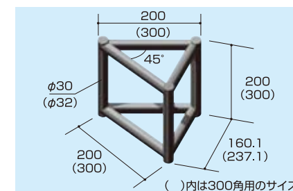
096-32 45°コーナー 200角用 095-34 45°コーナー 300角用
