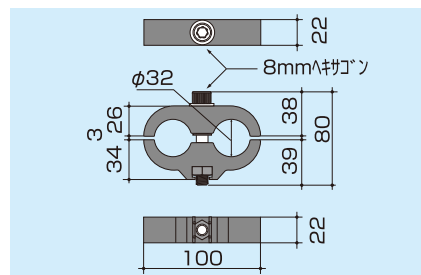
096-30 クランプ 200角用
