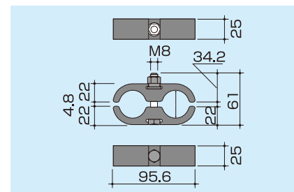
096-31 Cクランプ 200角・300角共用
