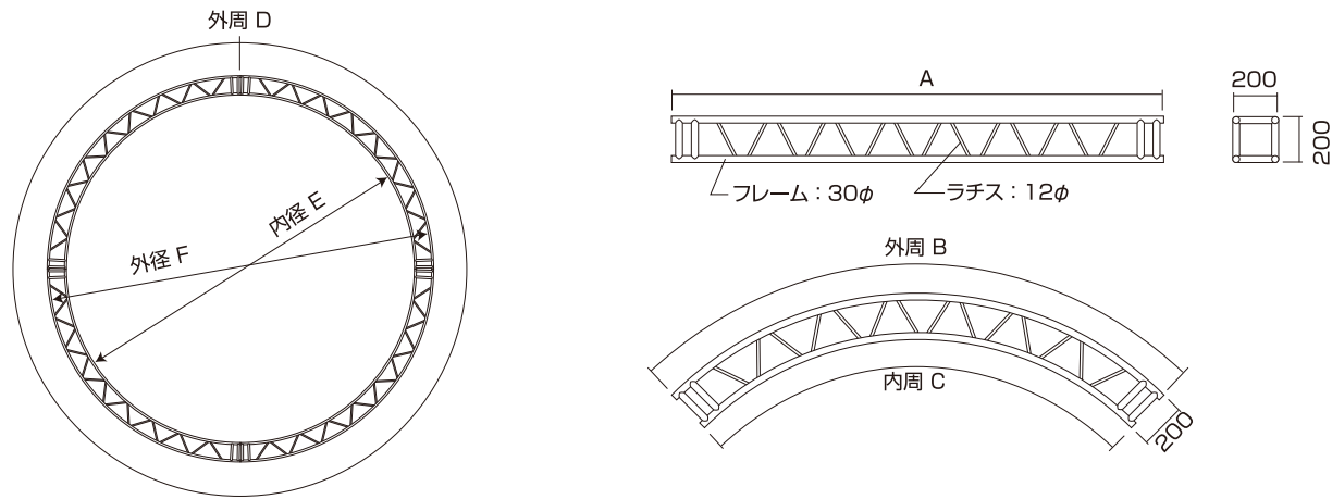
サイズ別外形寸法表
