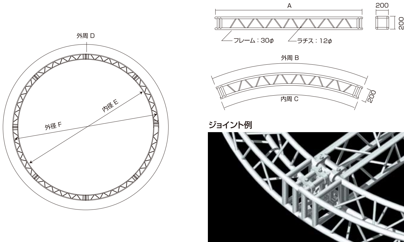
サイズ別外形寸法表
